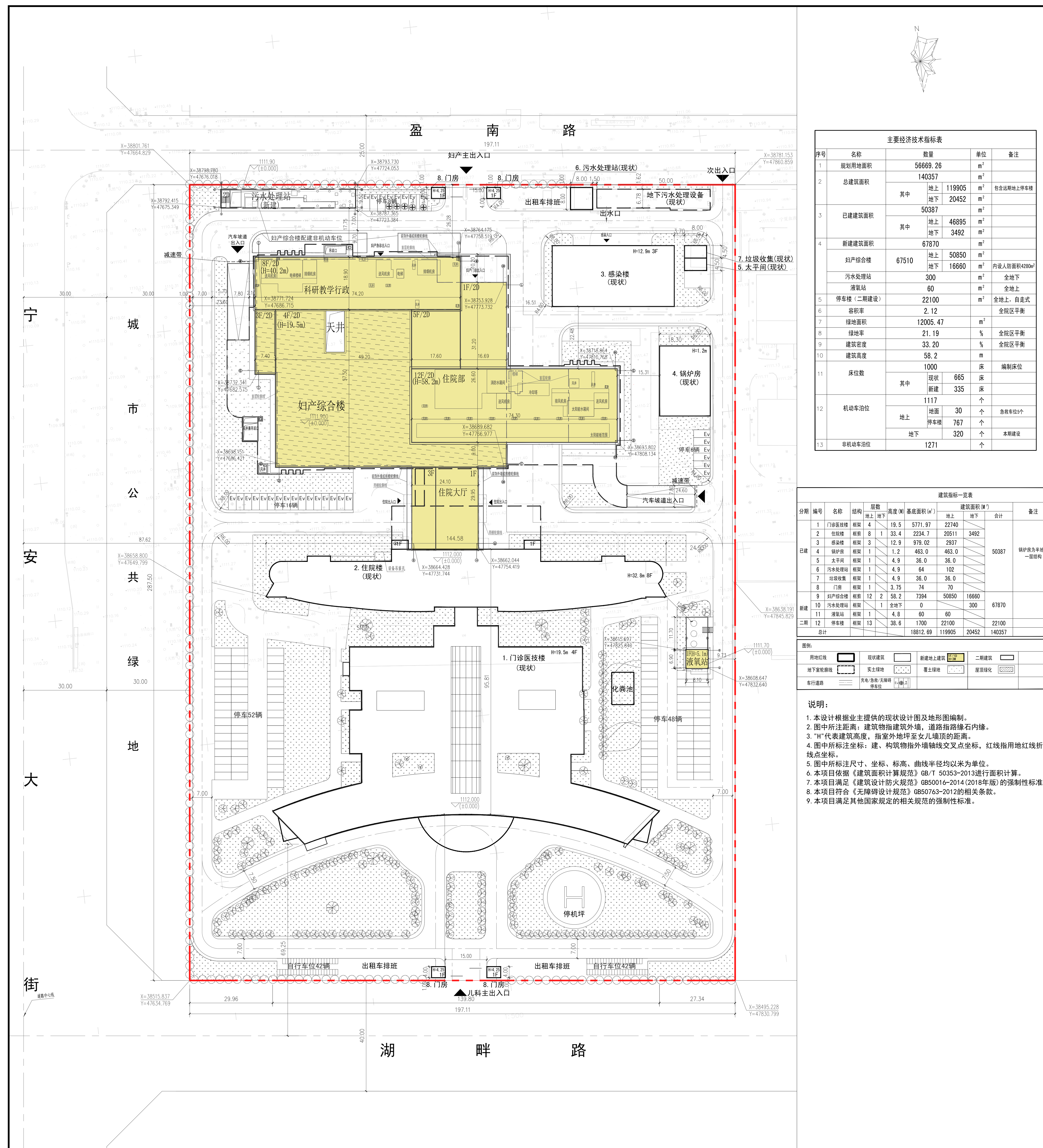
总平面图
