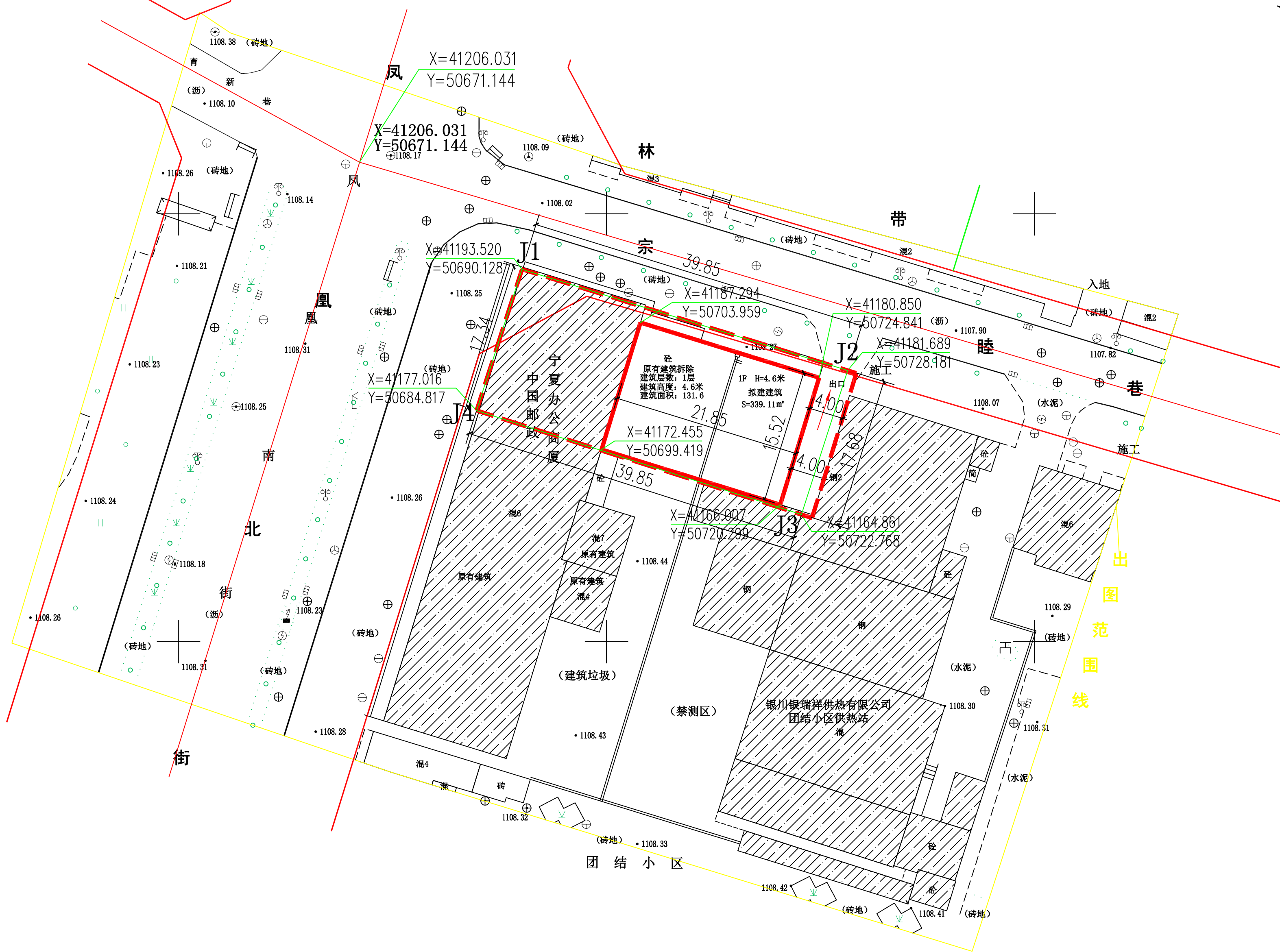
拟调整总平面图
